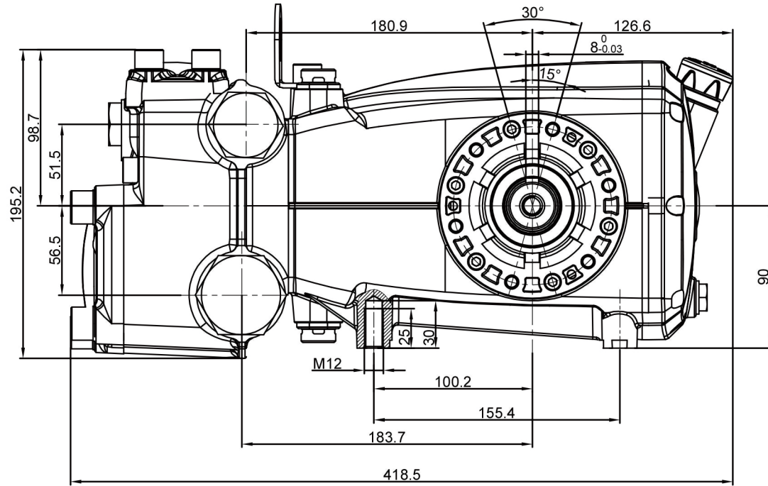
GT系列外形尺寸图
