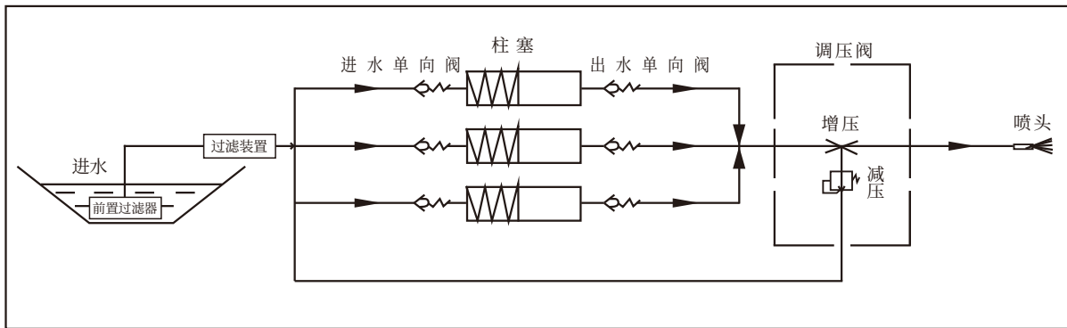
工作原理图
