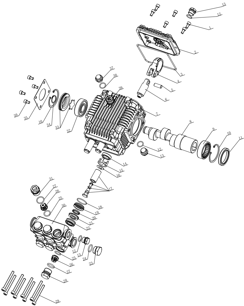
1、LB-C 分解图及明细表
