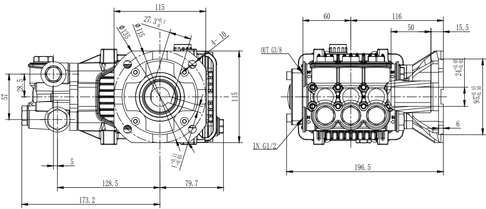
LB-F2 安装尺寸图
