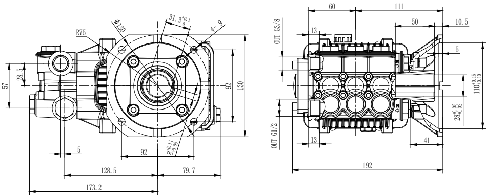
LB-F2 安装尺寸图
